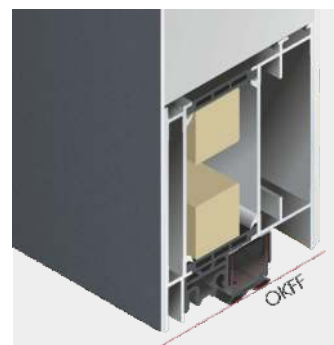
FP5 automatische Türabdichtung
