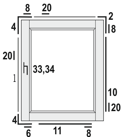
1-Flg. Fenster
