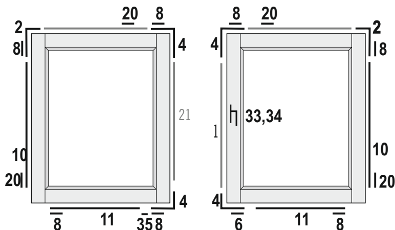
2-Flg. Fenster
