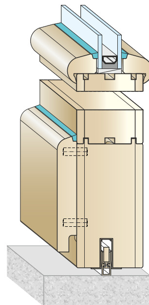
ALTERNATIVAUSFÜHRUNG SOFT (Glasleisten, Wetterschenkel) AV-07 Bodenprofil
