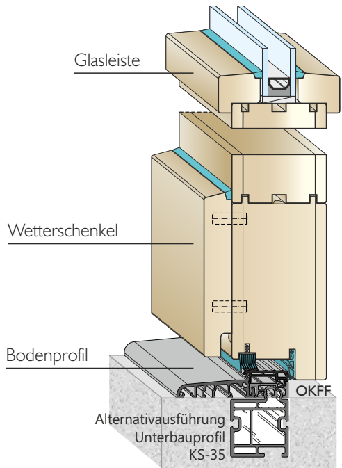
STANDARDAUSFÜHRUNG HH 68 KANTIGE (Glasleiste, Wetterschenkel) BKV 80 TB Bodenprofil
