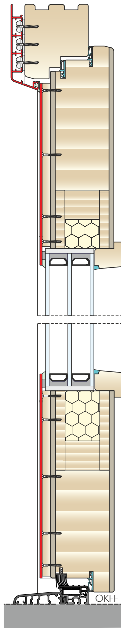
Serie TREND MODERN
