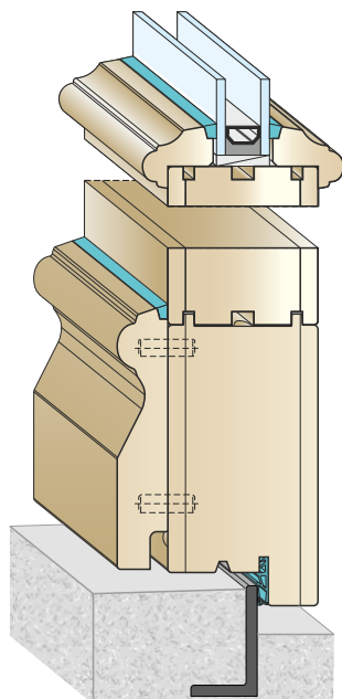
ALTERNATIVAUSFÜHRUNG PROFILIERTE (Glasleisten, Wetterschenkel) AV-02 Bodenprofil
