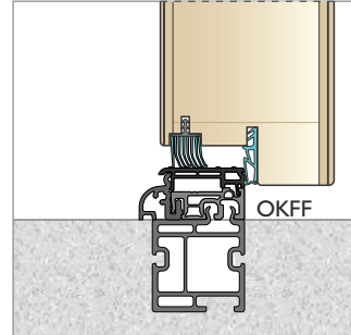
STANDARDAUSFÜHRUNG HH 80 BKV 40 TB Bodenprofil
