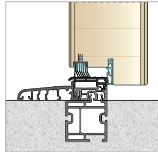
ALTERNATIVAUSFÜHRUNG HH 80 BKV 80 TB Bodenprofil
