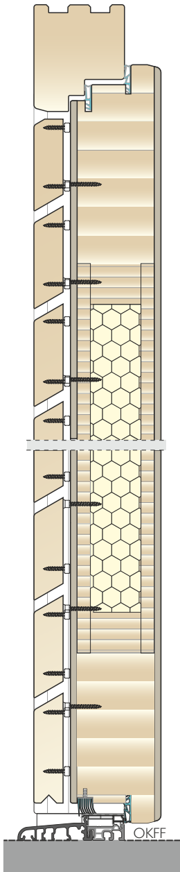
Serie TREND LINE
